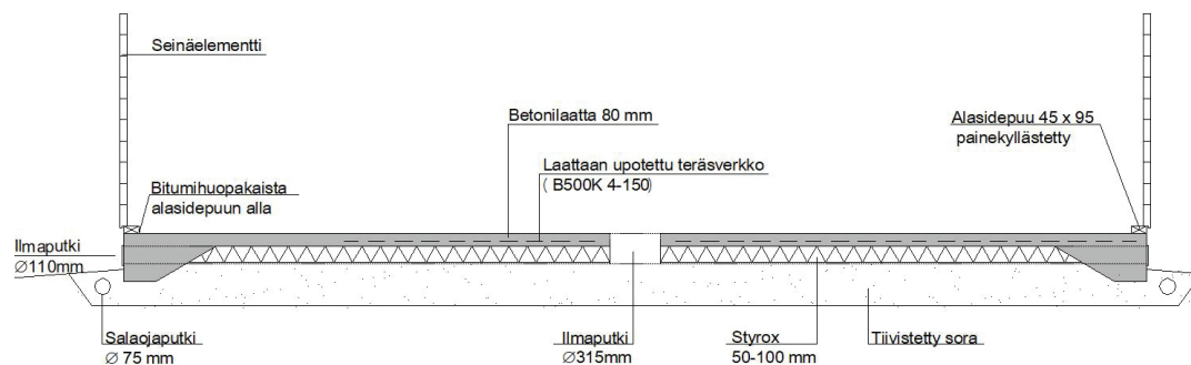
Perustukset Leikkaus A - A :
