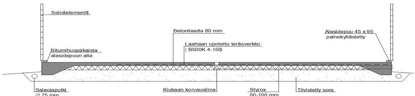
Perustukset Leikkaus A-A:
