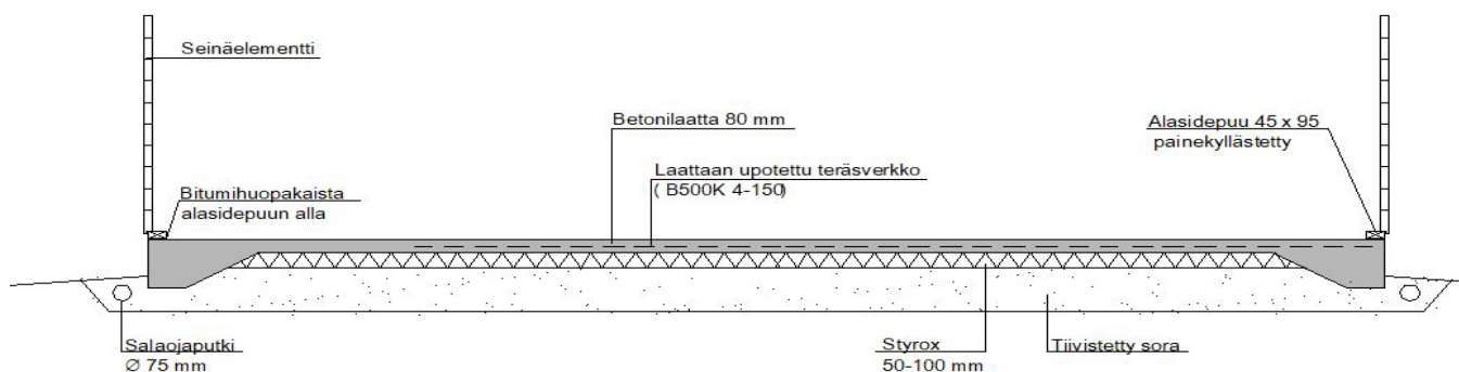
Perustukset Leikkaus A - A :
