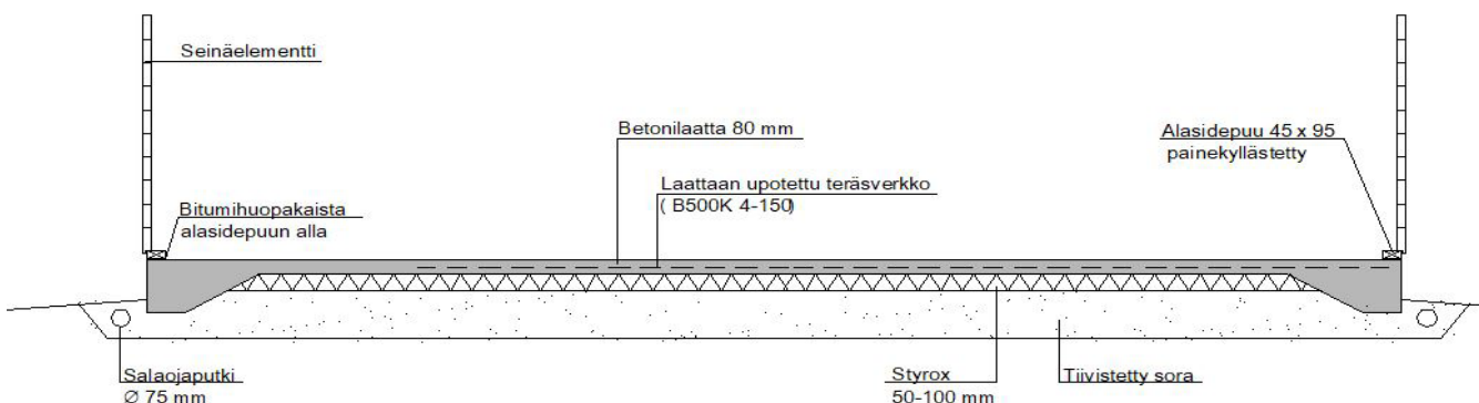
Perustukset Leikkaus A - A :
