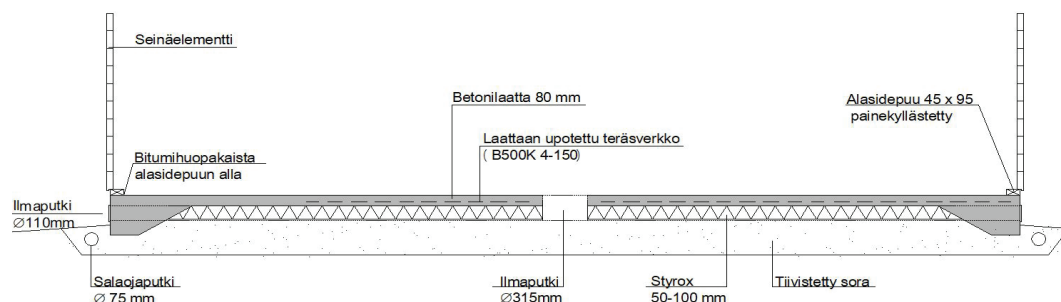
Perustukset Leikkaus A - A:
